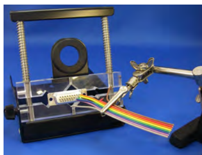
治具「てだすけ君」を使った固定
